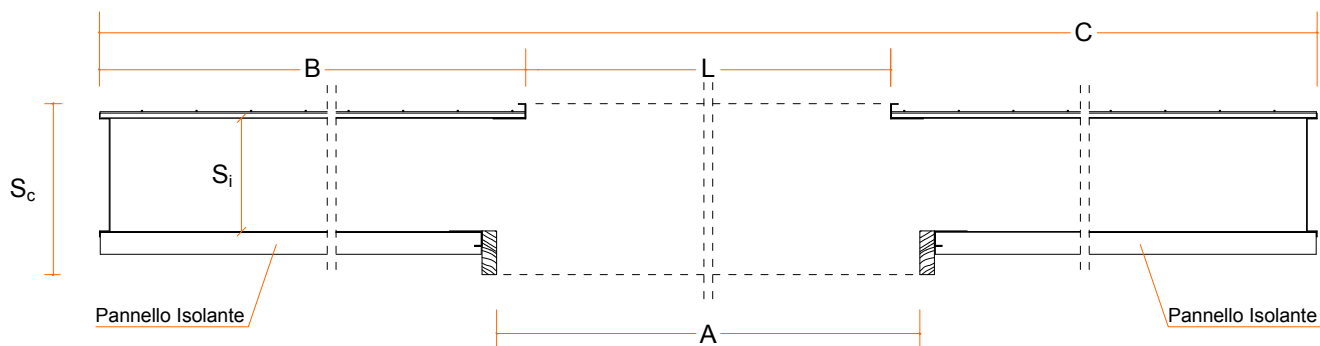
SEZIONE ORIZZONTALE
