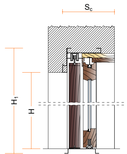
SEZIONE VERTICALE
