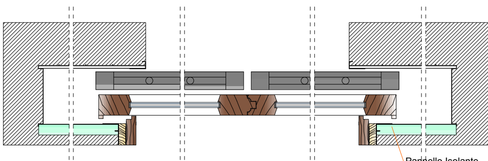
SEZIONE ORIZZONTALE
