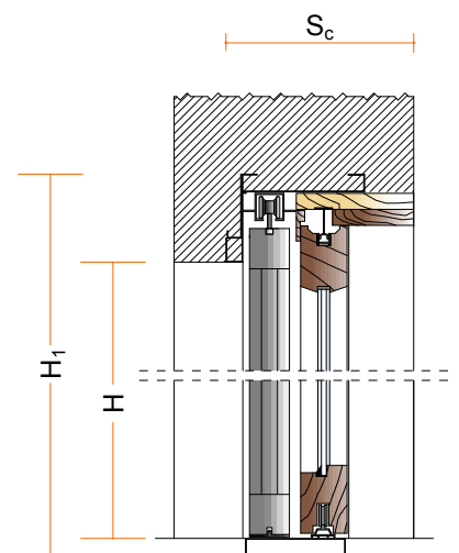
SEZIONE VERTICALE
