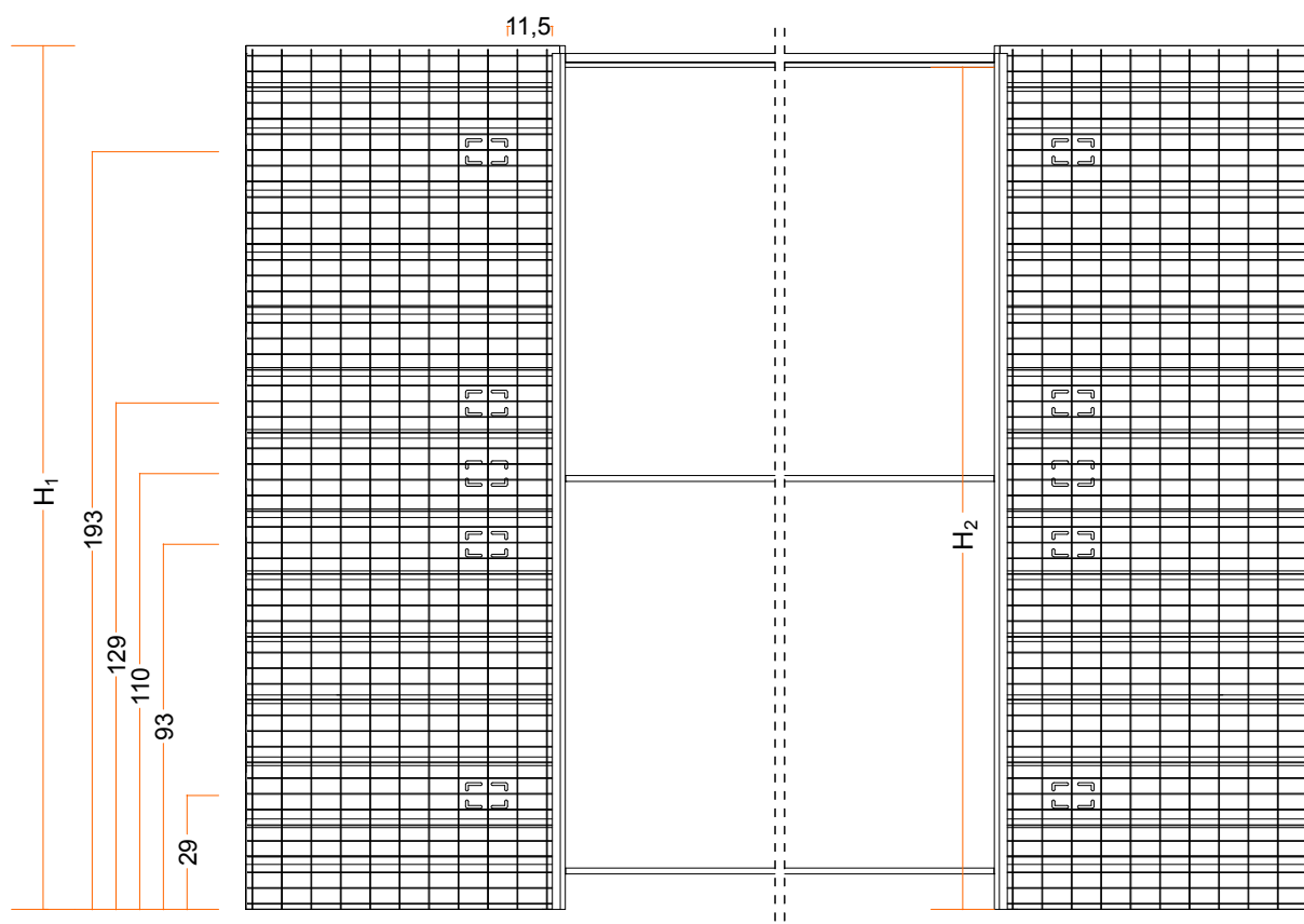
PROSPETTO
