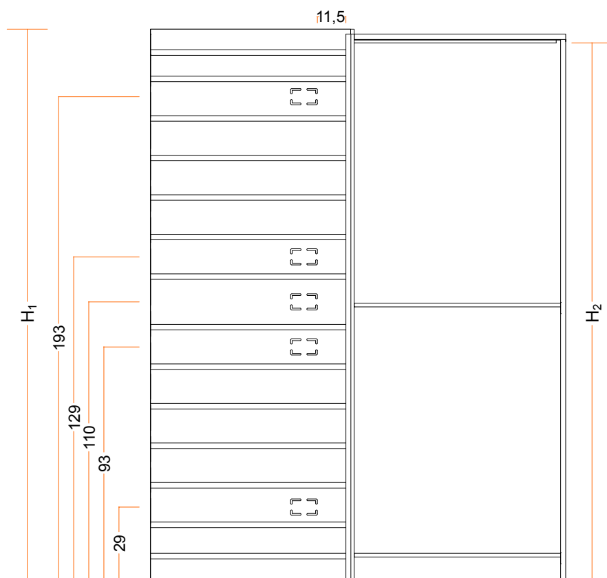
PROSPETTO
