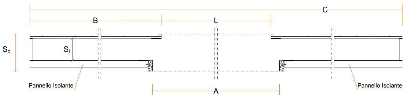
SEZIONE ORIZZONTALE
