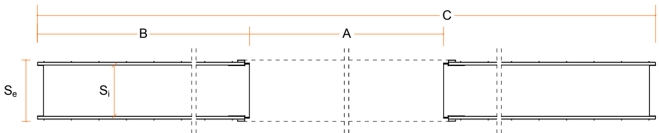
SEZIONE ORIZZONTALE
