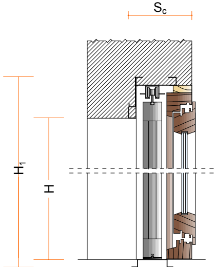
SEZIONE VERTICALE
