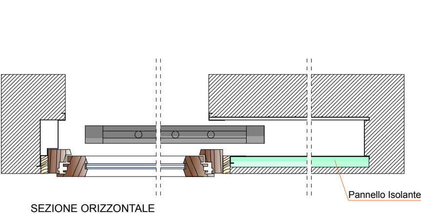
SEZIONE ORIZZONTALE
