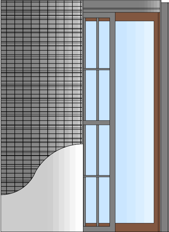
PROSPETTO ESTERNO
